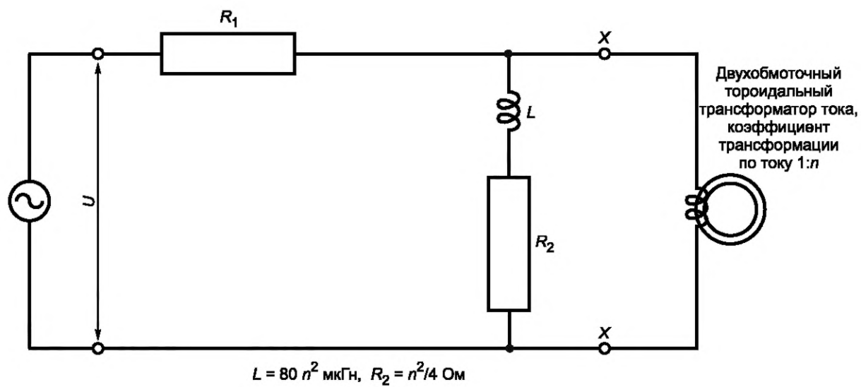
Рисунок В.4 — Выравнивающая цепь
