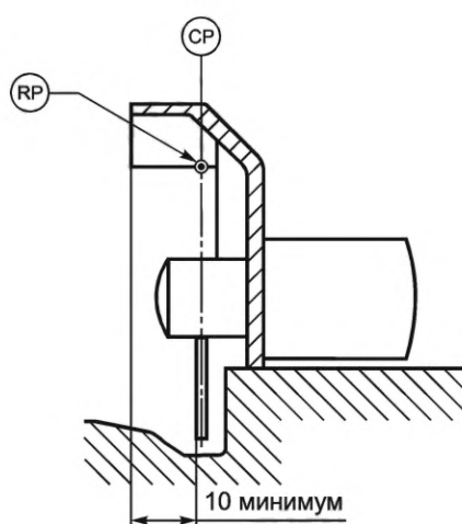
Рисунок 102a — Частичный разрез AA (только защита)
