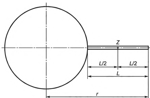
Рисунок 105а — Линия режущей нити
