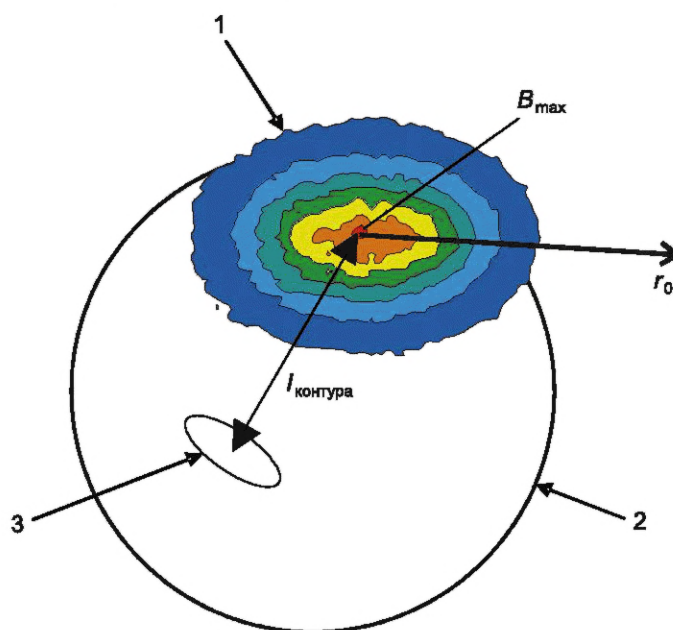
1 — измерение по касательной плоскости вокруг точки с максимальной интенсивностью; 2 — модель бытового электрического прибора в виде сферы; 3 — контур в качестве эквивалентного источника поля
