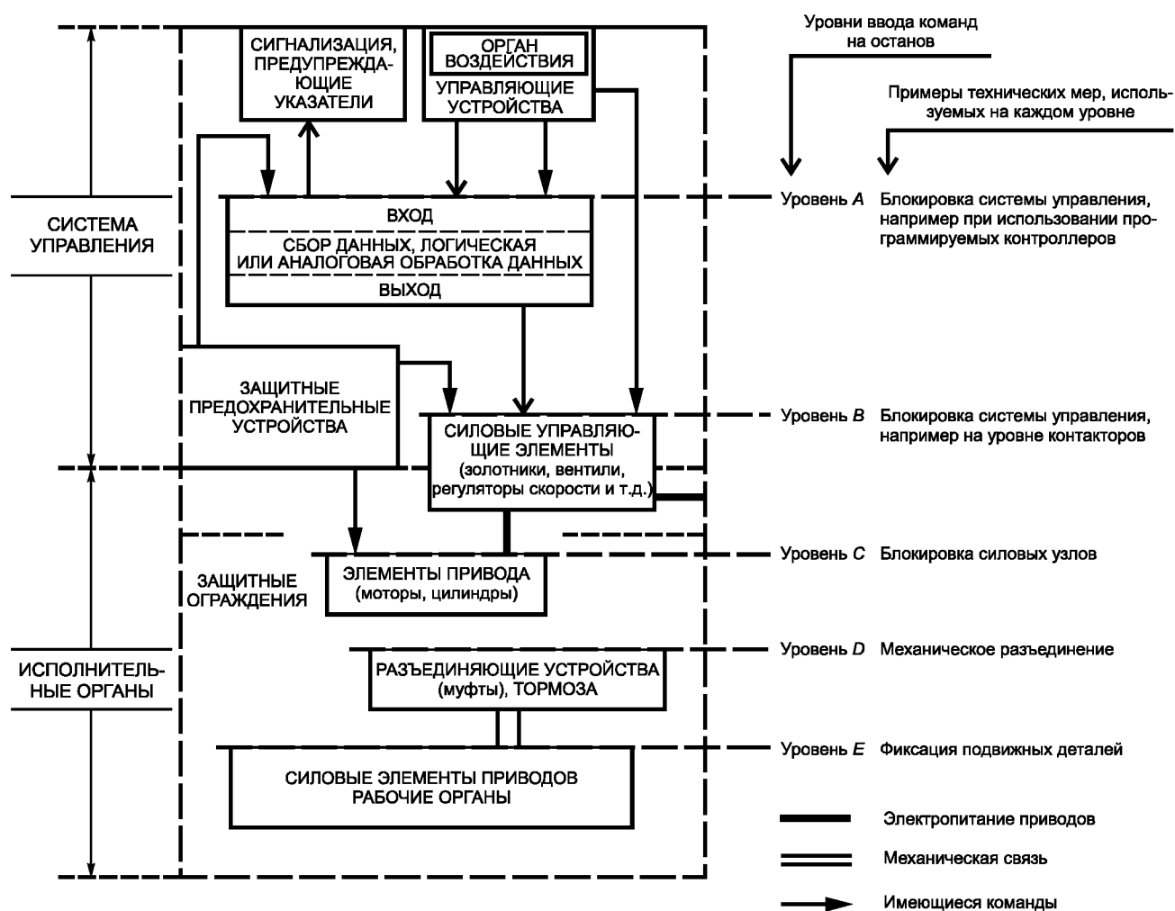
Рисунок 1 — Применение мер безопасности, кроме отвода или поглощения энергии, в порядке предупреждения непреднамеренного пуска машины (ГОСТ Р 51333; приложение А)
