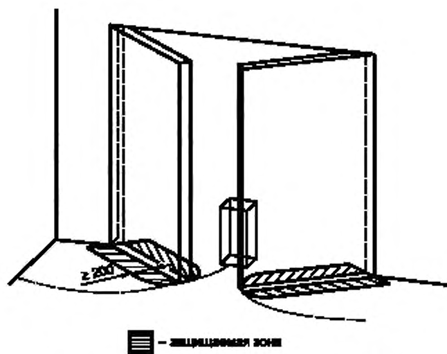
Рисунок ЕЕ.4 — Двустворчатый распашной дверной блок
