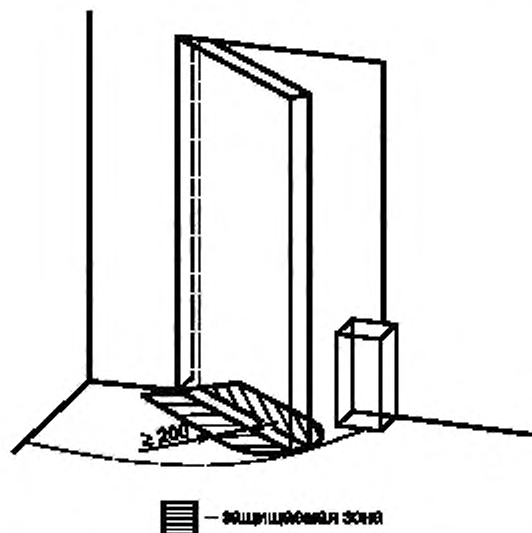
Рисунок ЕЕ.3 — Одностворчатый распашной дверной блок
