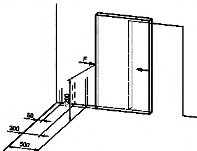
Рисунок II.1 — Одностворчатый раздвижной дверной блок
