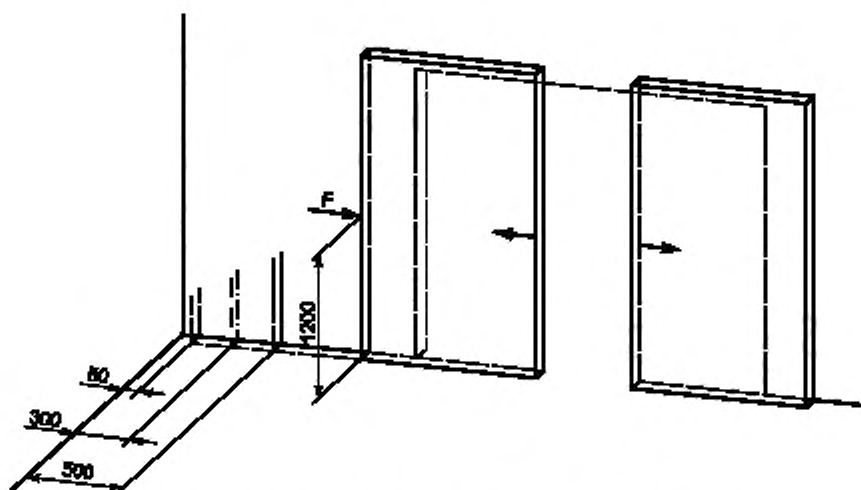
Рисунок II.2 — Двустворчатый раздвижной дверной блок
