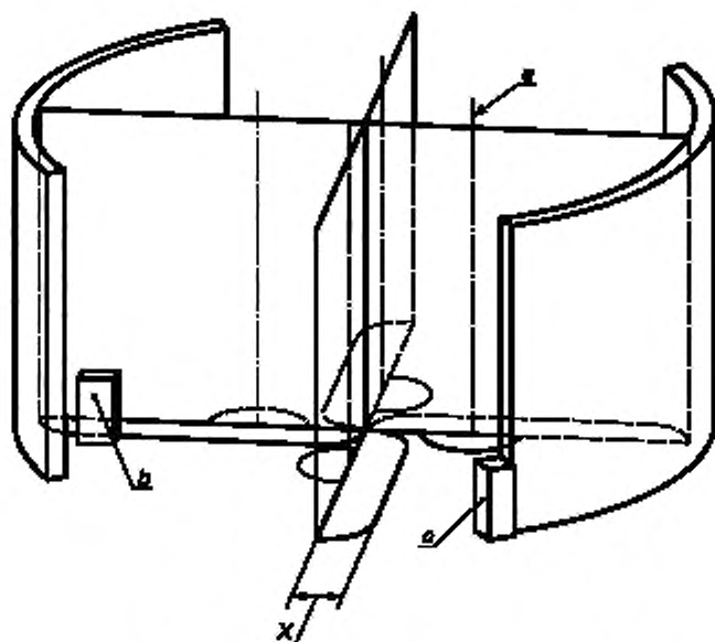
Рисунок ЕЕ.7 — Вращающиеся дверные блоки, три полотна
