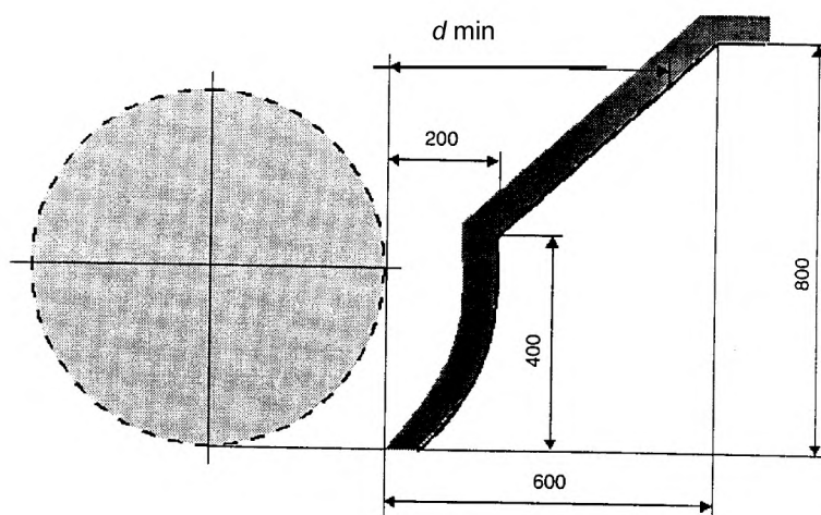
Рисунок 4 – Заднее защитное ограждение с шарниром
