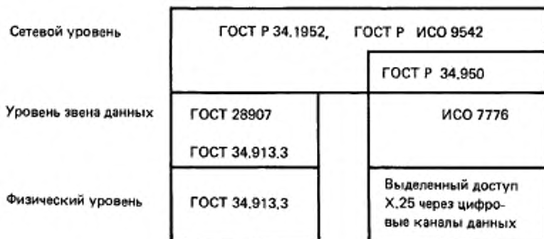
Рисунок 2 — Стек протоколов профиля
