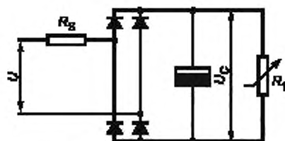
Рисунок М.4 — Эталонная нелинейная нагрузка
