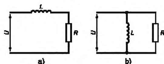
Рисунок М.2 — Эталонная активно-индуктивная нагрузка
