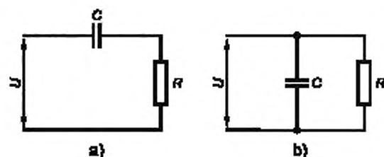
Рисунок М.3 — Эталонная активно-емкостная нагрузка
