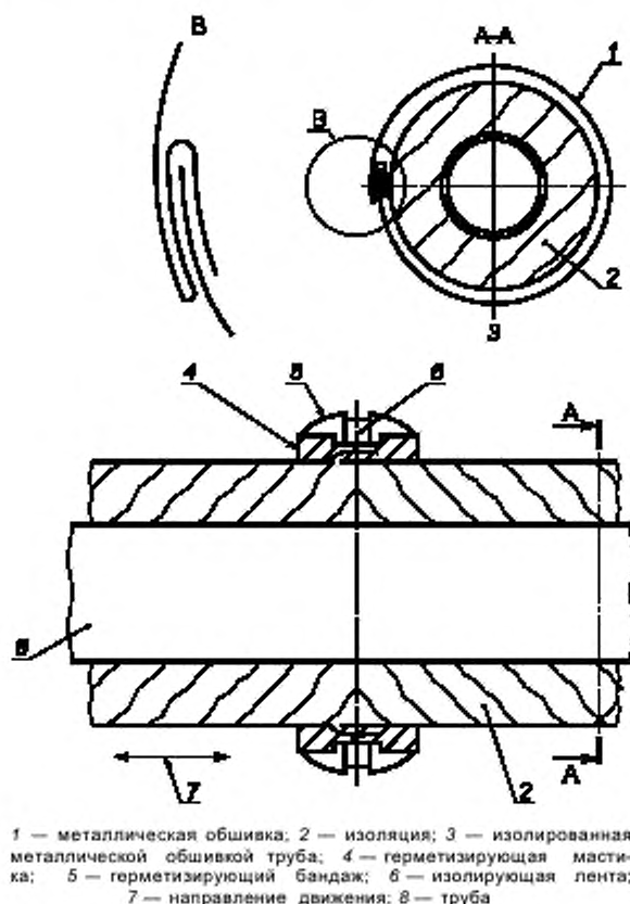
Рисунок 1 — Теплоизоляция: установка климатического барьера
