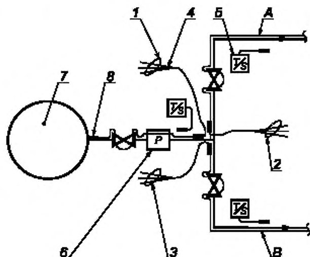
А — труба А; В — труба В; 1 — цель № 1; 2 — цель № 2; 3 — цель № 3; 4 — заделка холодного конца; 5 — температурный датчик; 6 — насос; 7 — обогреваемый резервуар; 8 — заделка горячего конца
