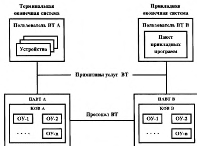
Рисунок 2 — Объекты управления в модели протокола ВТ
