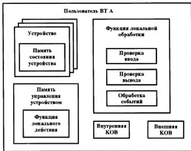
Рисунок 3 — Структура терминального пользователя ВТ
