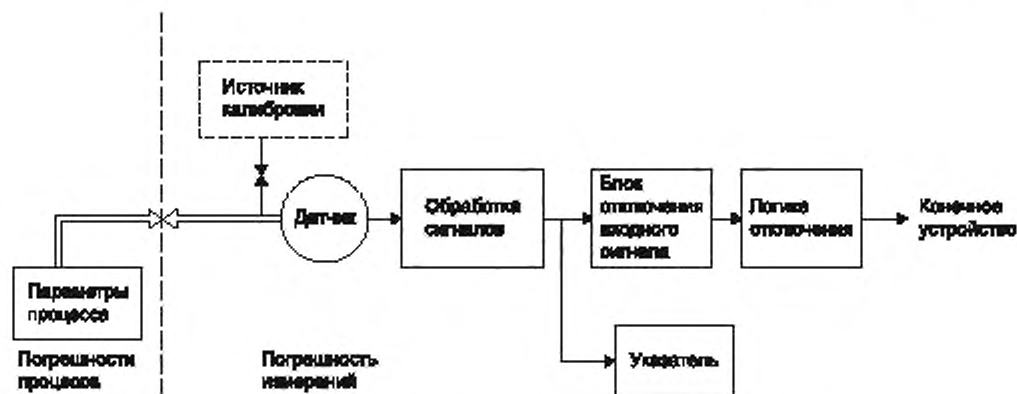
Рисунок 2 — Погрешности процесса и измерительных приборов
