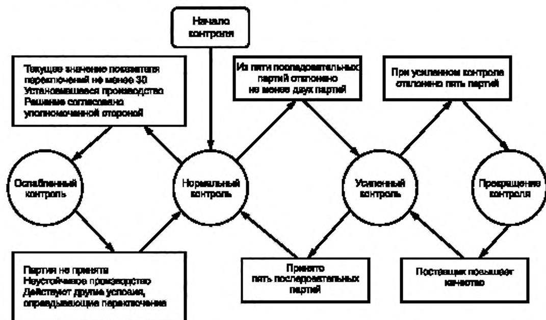
Рисунок 1 — Схема правил переключения (см. 10.3)
