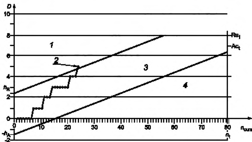
1 — зона отклонения; 2 — прекращение контроля; 3 — зона неопределенности; 4 — зона приемки
