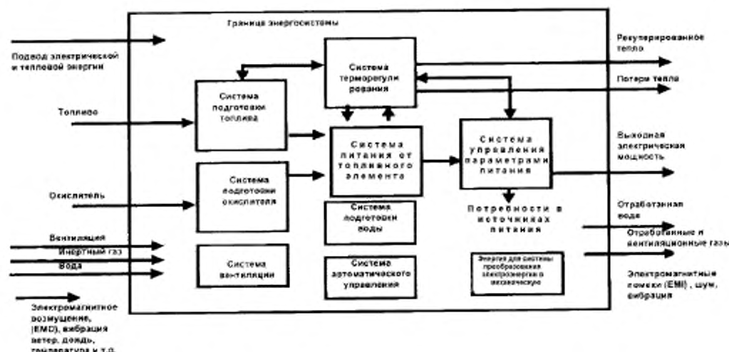
Рисунок 1 — Компоненты энергоустановки на топливных элементах
