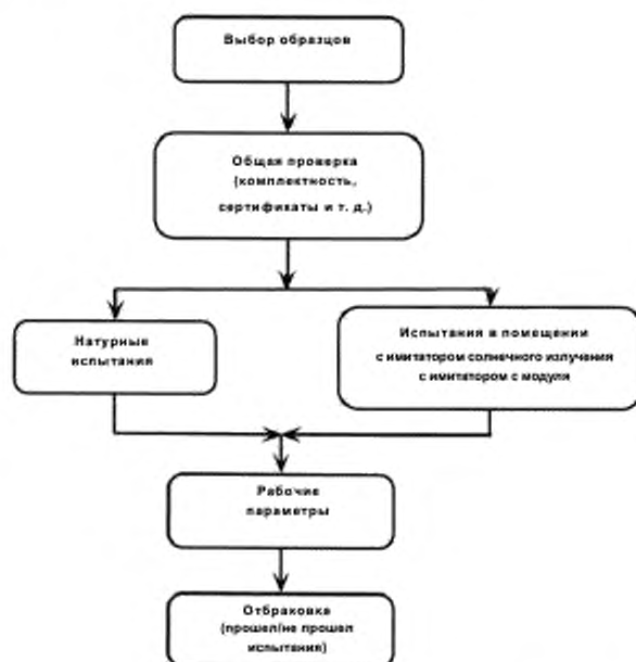
Рисунок 1 – Порядок проверки работоспособности автономной фотоэлектрической системы
