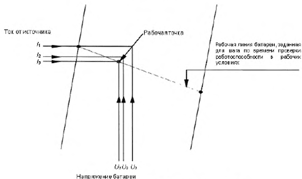
Рисунок С.4 — Итерационный процесс уточнения тока
