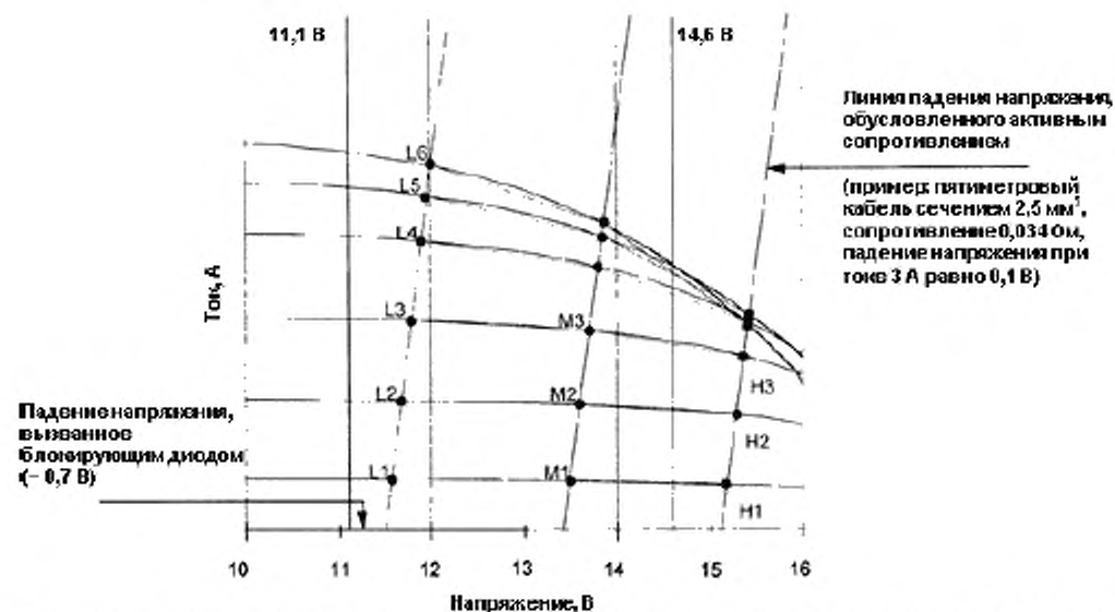
Рисунок С.3 — Пример аппроксимации ВАХ фотоэлектрической батареи с помощью набора рабочих линий батареи (АБ 12 В)
