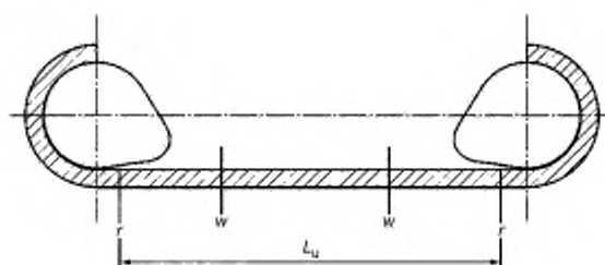
L_u — эффективная длина, измеренная без нагрузки; г — ограничительные метки для стандартного испытания; w — базовые метки для стандартного испытания
