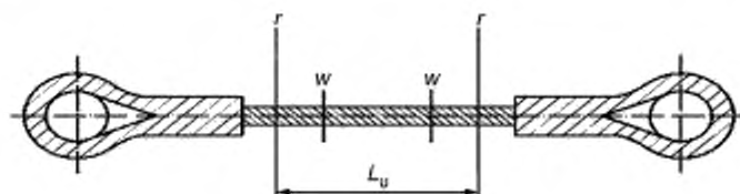
L_u — эффективная длина, измеренная без нагрузки; г — ограничительные метки для стандартного испытания; w — базовые метки для стандартного испытания
