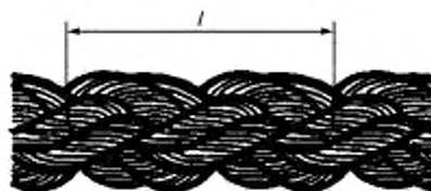
l — один шаг плетения 8-прядного плетеного каната
