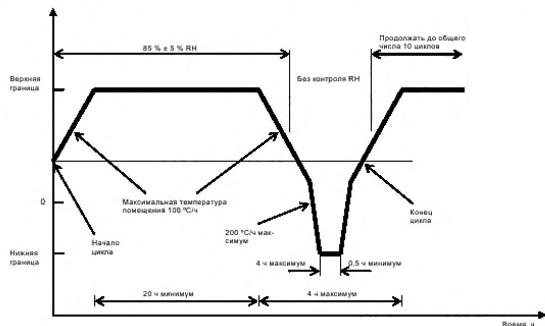
Рисунок 5 — Испытание на стойкость к влажности и низким температурам
