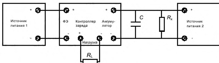
Рисунок 3 — Схема проверки без подключения измерительных приборов
