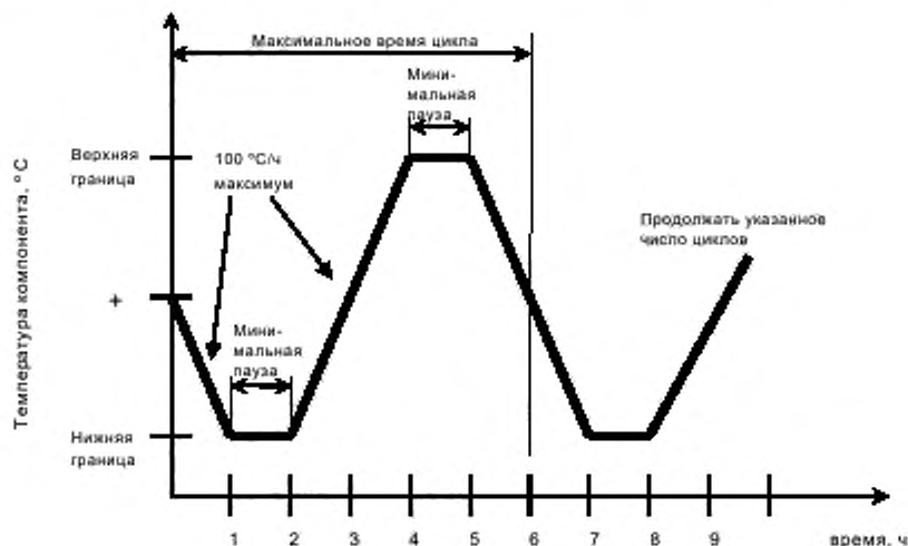
Рисунок 4 — Термоциклирование
