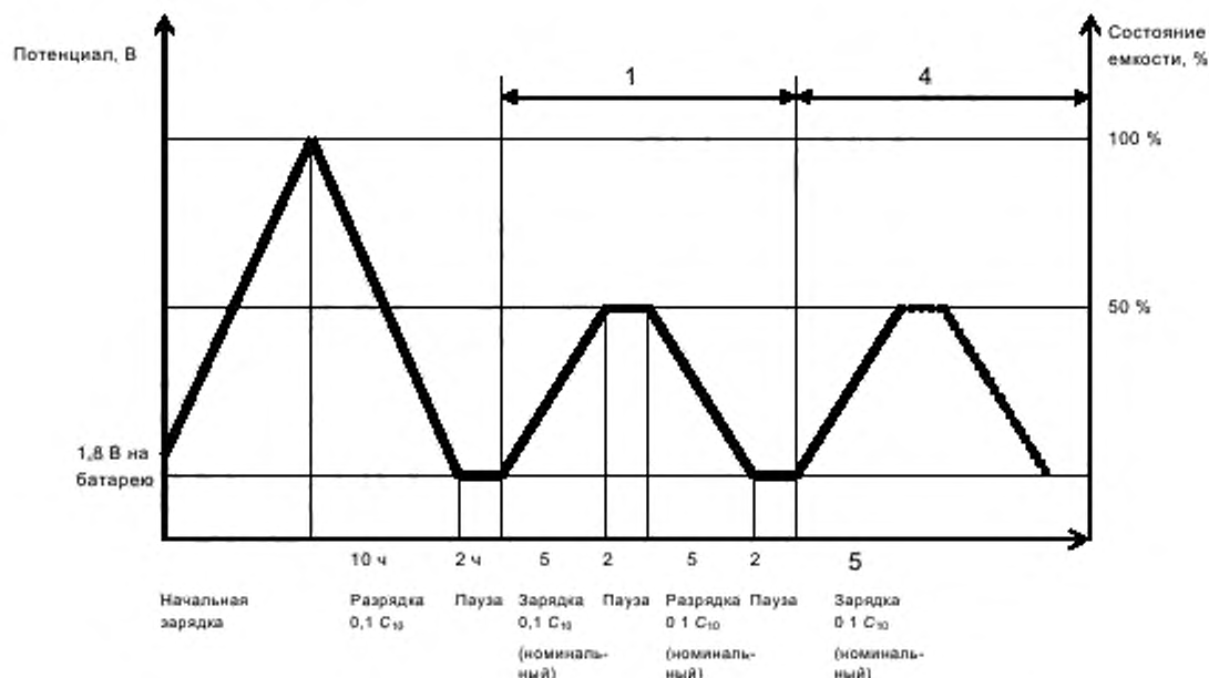
Рисунок 2 — Циклические условия эффективности метода испытаний
