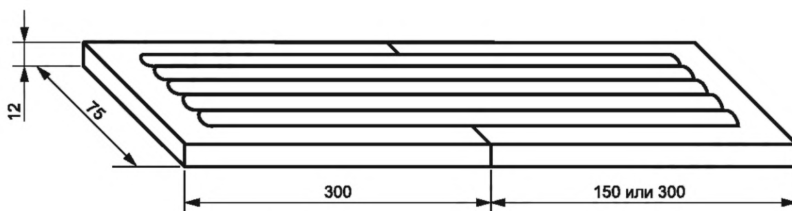
Рисунок 1 — Испытательный образец
