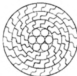
б) трехжильный провод, скрученный из профилированных проволок типа AxF/Sxy
