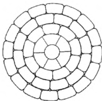
а) трехжильный провод, скрученный из профилированных проволок типа AxF/Sxy
