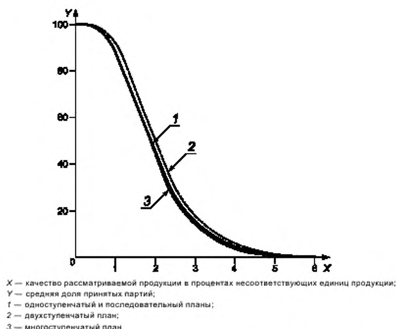
Рисунок 4 — Кривые операционных характеристик одноступенчатого, двухступенчатого, многоступенчатого и последовательного планов выборочного контроля
