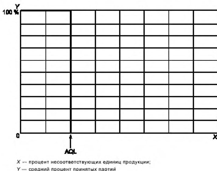
Рисунок 3 — Идеальная кривая оперативной характеристики
