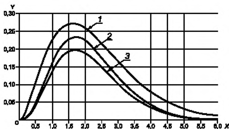
X — процент несоответствующих единиц продукции процесса; Y — вероятность превышения среднего объема выборки одноступенчатого контроля
