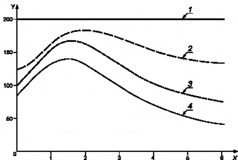
X — качество рассматриваемой продукции в процентах несоответствующих единиц продукции, 100р; Y — средний объем выборки; 1 — одноступенчатый план; 2 — двухступенчатый план; 3 — многоступенчатый план; 4 — последовательный план
