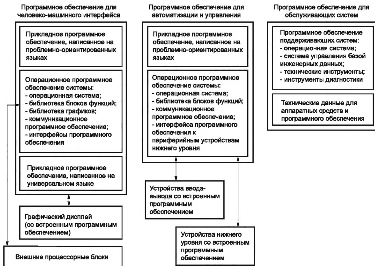
Рисунок 1 — Типичные части ПО в компьютерных СКУ
