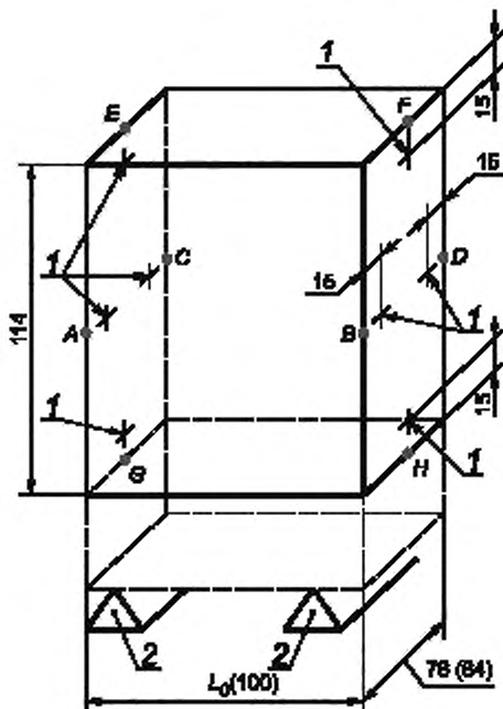
Рисунок 1 — Места измерений и установка образцов в печи
