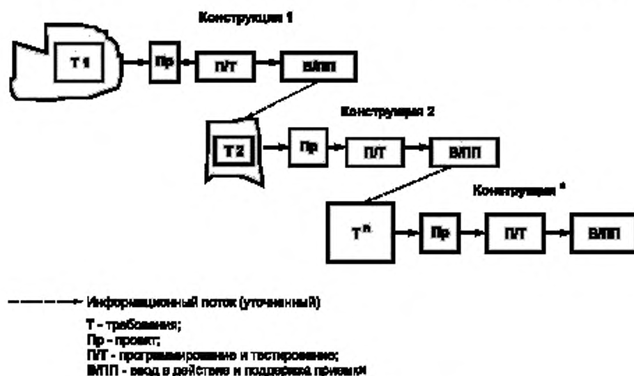
Рисунок С.3 — Пример эволюционной модели
