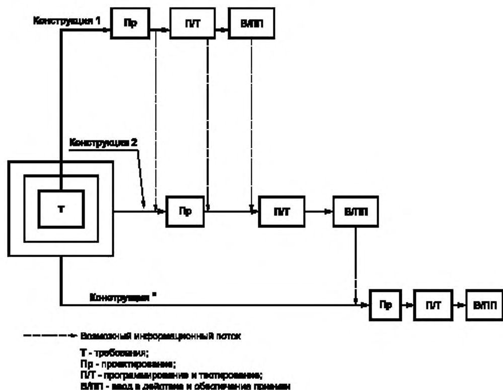
Рисунок С.2 — Пример инкрементной модели
