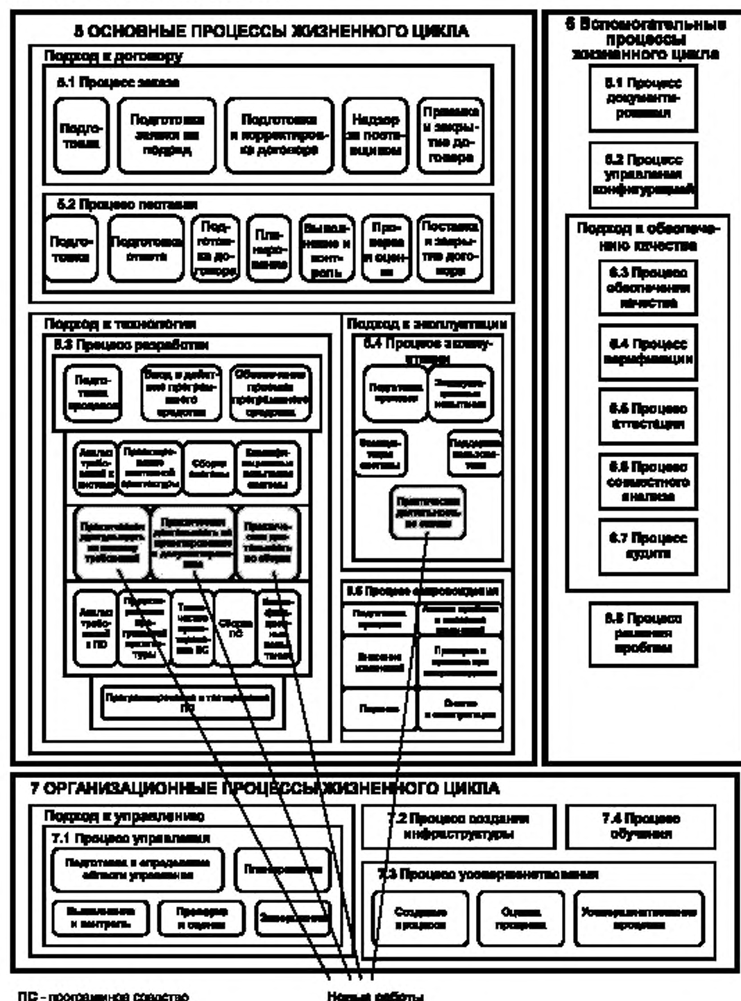
Рисунок D.1 — Пример адаптации к практической деятельности
