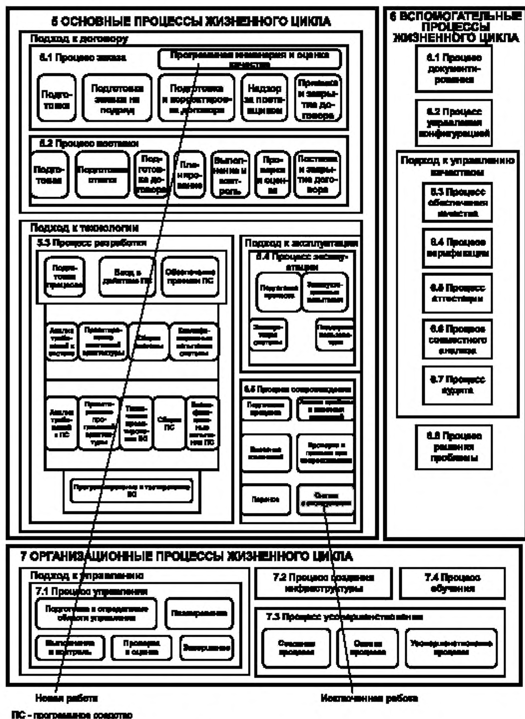
Рисунок D.4 — Пример адаптации сопровождения
