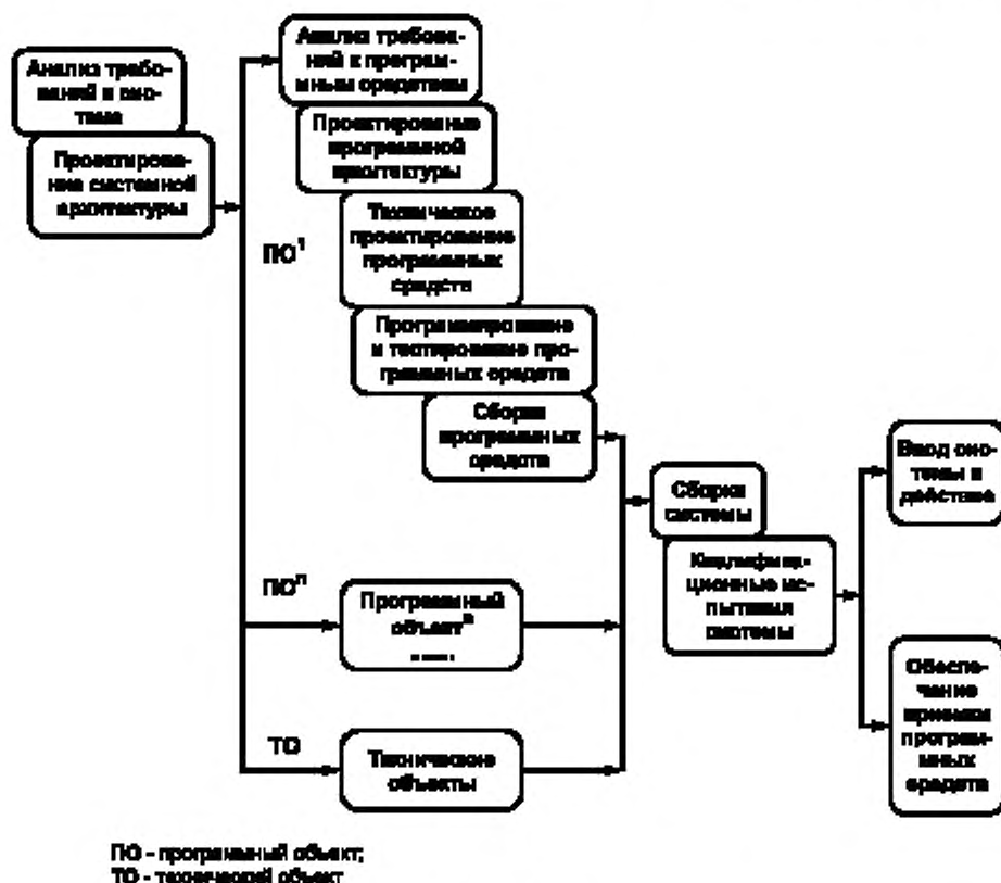
Рисунок С.1 — Пример каскадной модели
