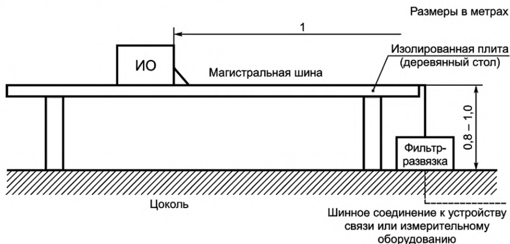
Рисунок СС.10 — Вид сбоку 1
