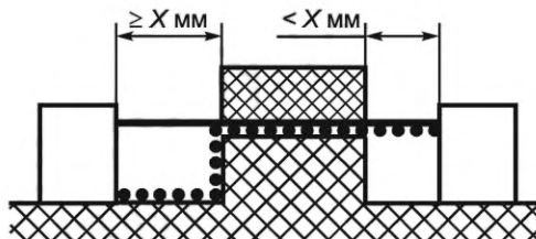
Рисунок ВВ.6 — Нецементированный стык с широкой канавкой
