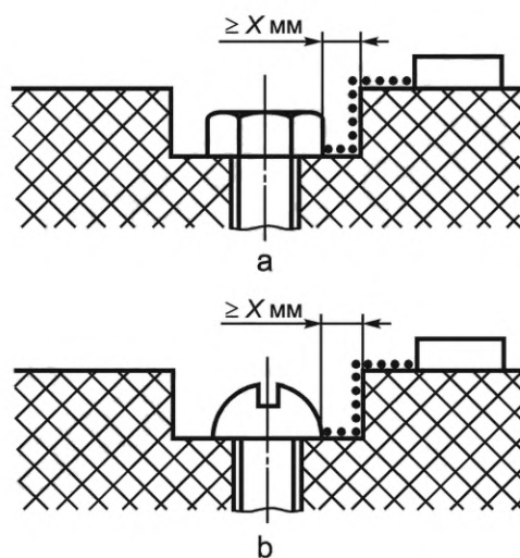
Рисунок ВВ.9 — Узкая выемка
