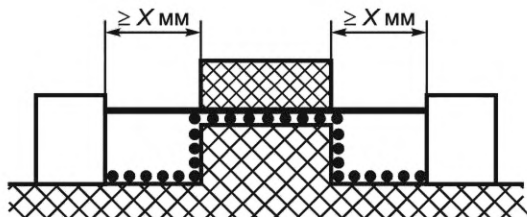
Рисунок ВВ.5 — Нецементированный стык с узкой канавкой
