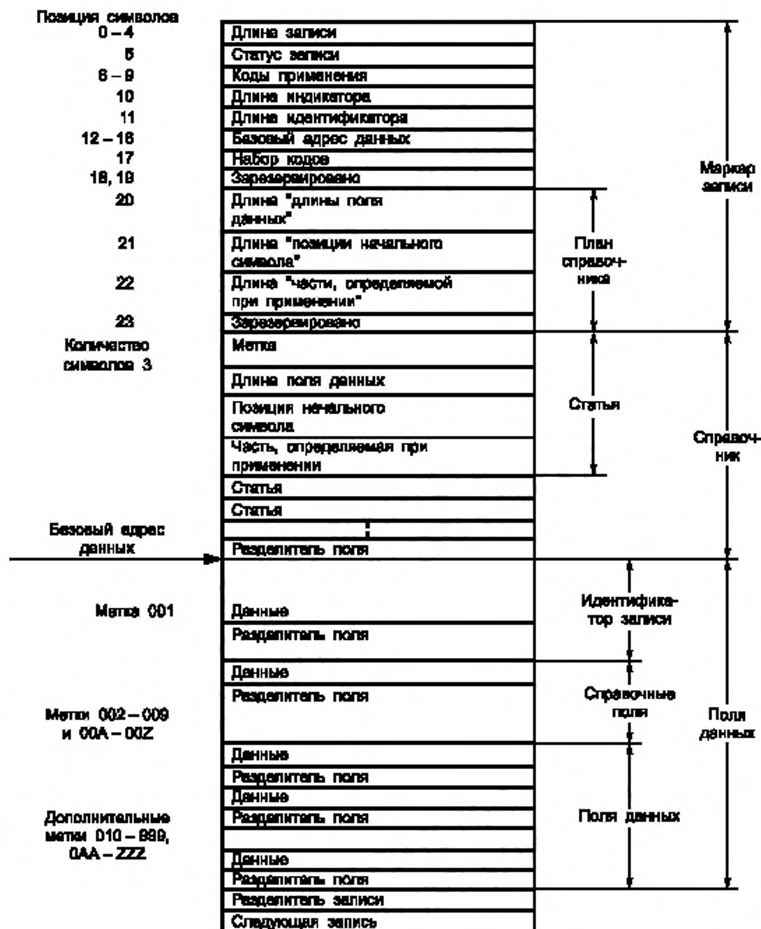
Рисунок 2 — Структура записи
