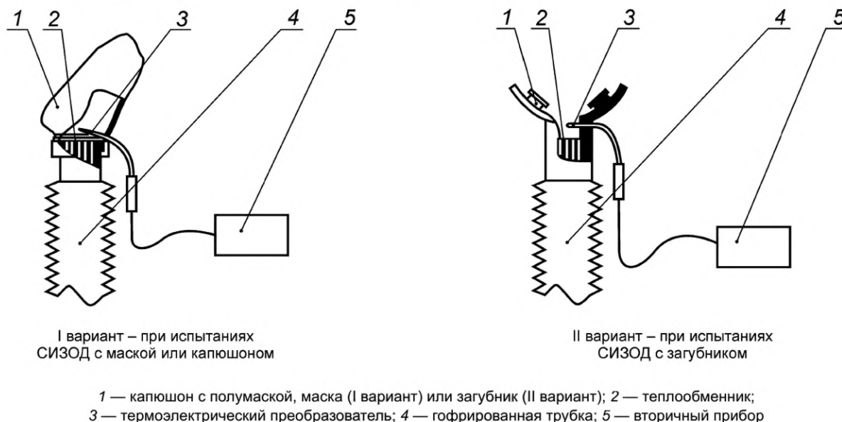
Рисунок 1 — Принципиальная схема измерения температуры вдыхаемой ГДС
