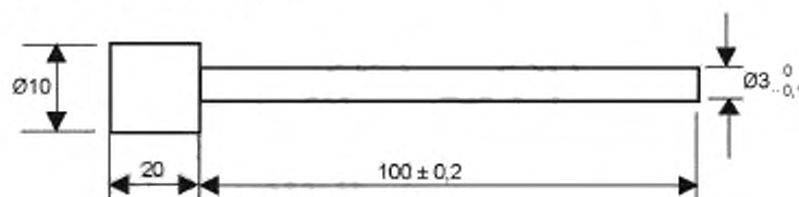
Рисунок 101 — Испытательный прут для скрытой блокировки
