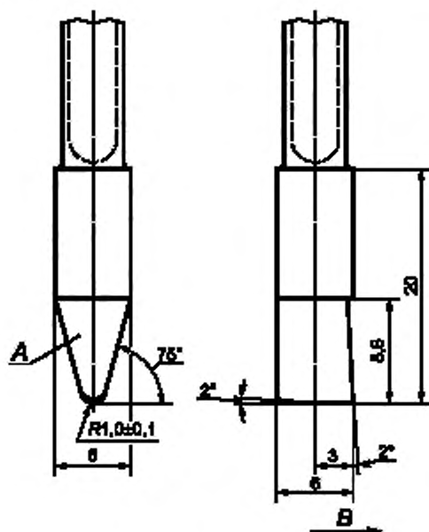
A — твердосплавный наконечник типа K10; B — направление движения
