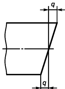
Рисунок 3 — Контроль перпендикулярности реза
