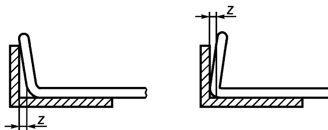
Рисунок 2 — Определение наклона боковой стороны
