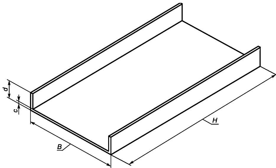
Рисунок 1 — Размеры закаленного натрий-кальций-силикатного профильного безопасного стекла
