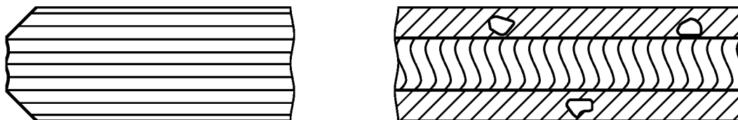
Рисунок 6 — Притупленная кромка (есть необработанные участки)
