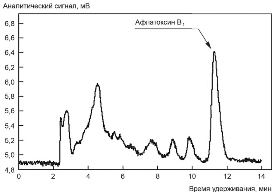
Рисунок А.1 — Пример типичной хроматограммы при определении афлатоксина В 1 в продукте для питания детей раннего возраста с применением очистки экстракта на иммуноаффинной колонке. Содержание афлатоксина В 1 — 0,1 мкг/кг
