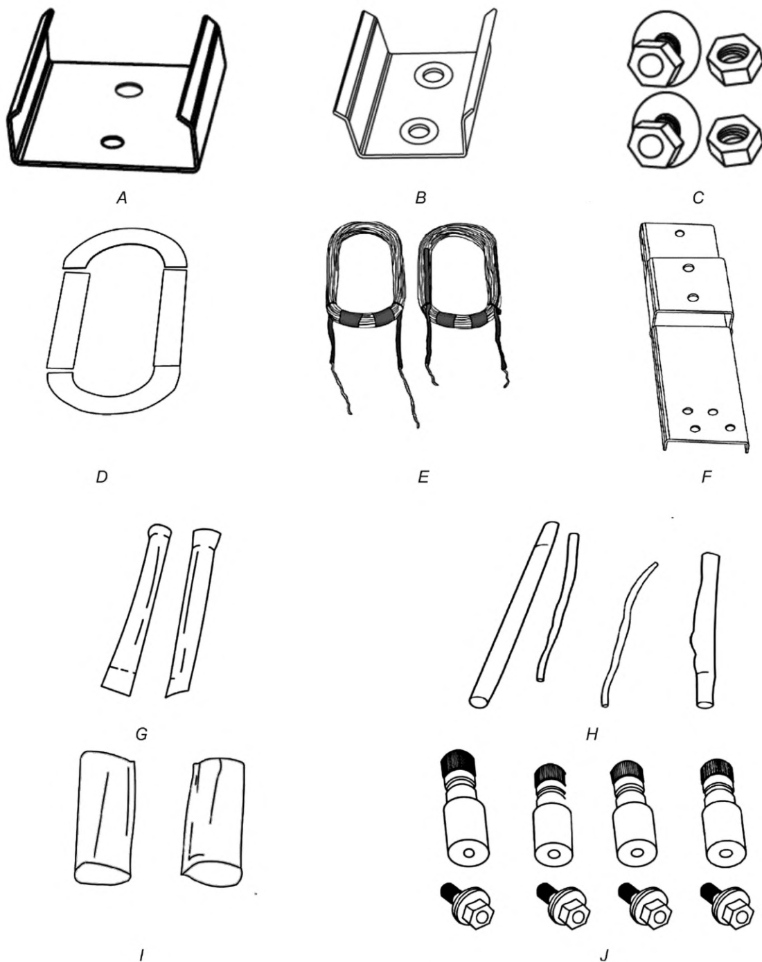
А — наружный слот пластины; В — внутренний слот пластины; С — болты, гайки и шайбы; D — фазная изоляция; Е — бифилярные катушки с произвольной намоткой; F — латунная рама; G — пазовые клинья; H — защитные изолирующие трубки; I — пазовая изоляция; J — клеммы и изоляторы
