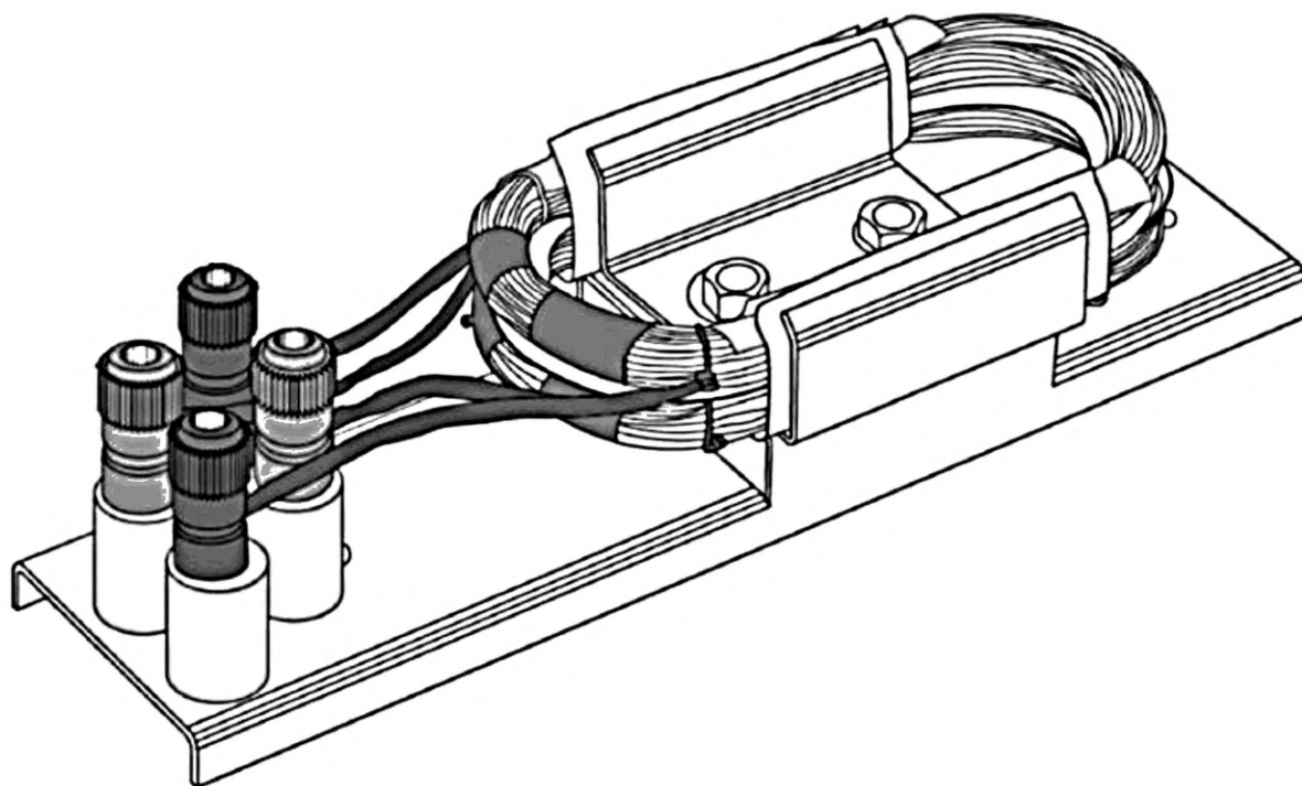
Рисунок ВВ.2 — Полностью собранная модель motorette
