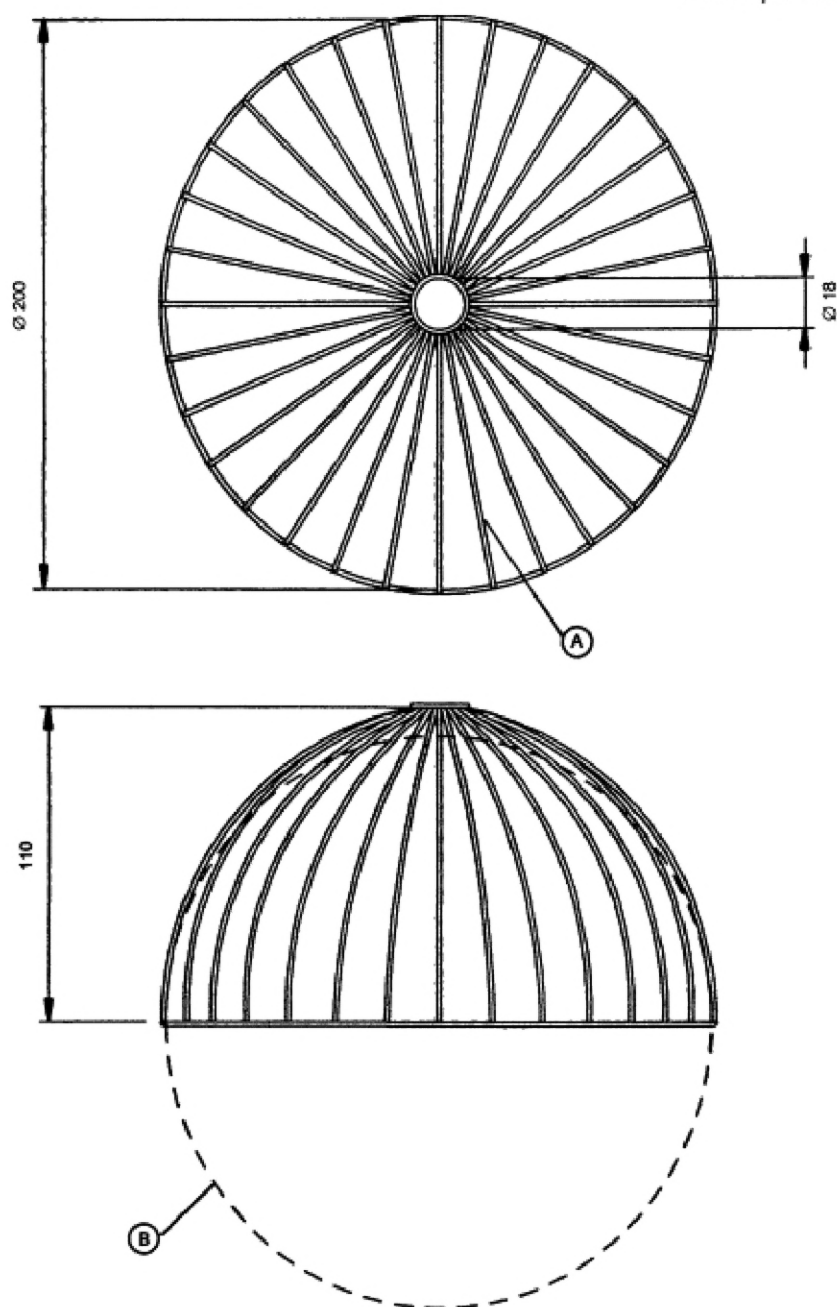
Рисунок 101 — Проволочный каркас
