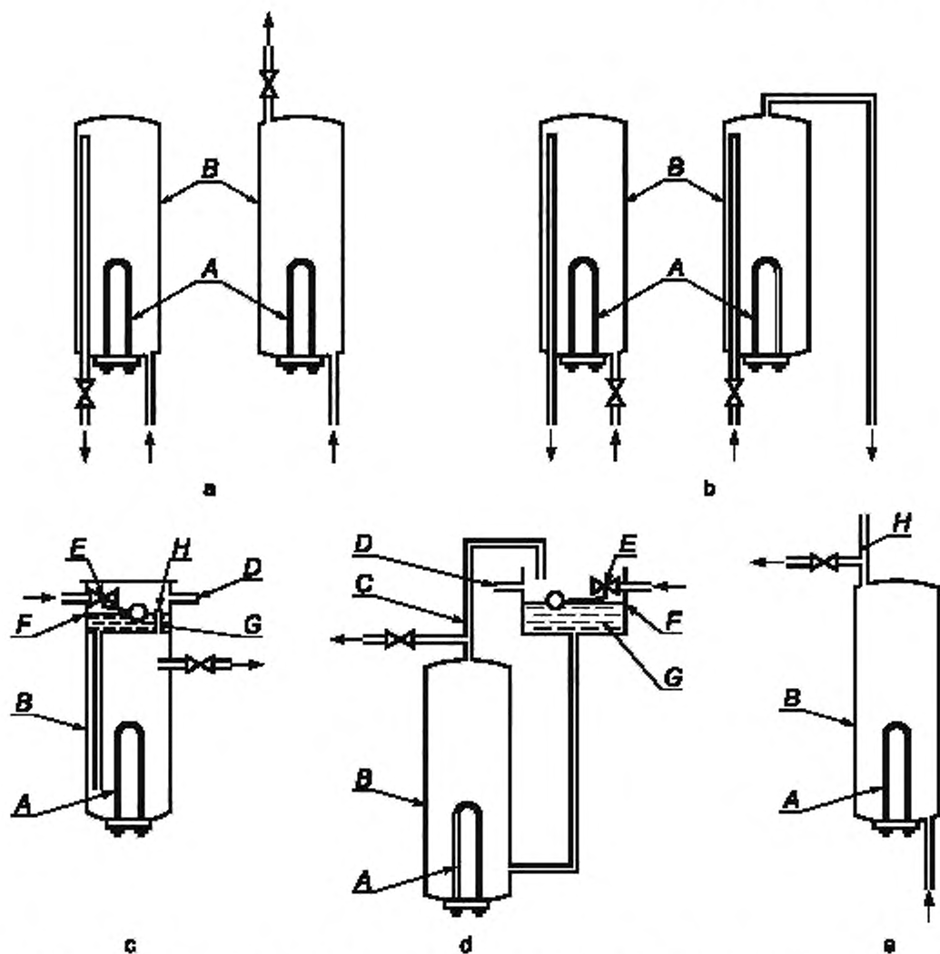
A — нагревательный элемент; B — бак; C — выходная труба; D — труба расширения; E — шаровый клапан; F — уровень воды; G — резервуар; H — вентиляционная труба
