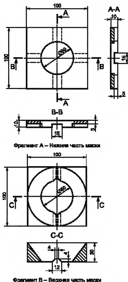
Рисунок 113а — Детальный чертеж маски
