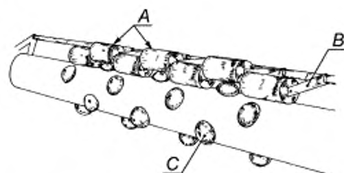
А — цилиндр; В — кронштейн цилиндра; С — сферы из монолитной резины
