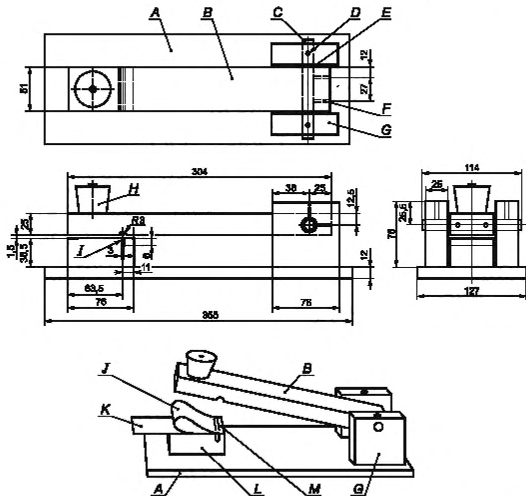
А — основание; В — рычаг; С — неплотно пригнанный штифт; D — уплотненное смазочное отверстие; E — механически обработанная шайба; F — отверстие с внутренней резьбой для установочных винтов; G — опора рычага; H — ручка; I — паз; J — образец; K — картон; L — опора; M — скобы
