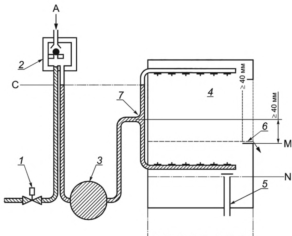
1 — электромагнитный клапан; 2 — динамическое устройство предотвращения противотока; 3 — нагреватель; 4 — ополаскивающая консоль; 5 — обычный сливной патрубок; 6 — переполнение в ненормальном режиме работы; 7 — точка разветвления; А — впускной воздушный клапан; С — критический уровень воды; М — максимальный уровень воды; N — нормальный уровень воды
