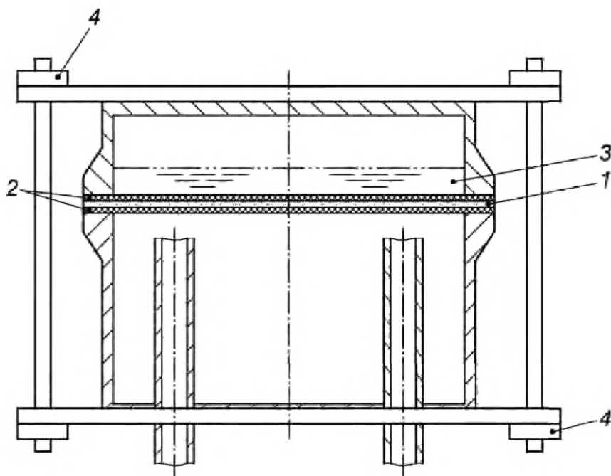
1 — испытуемая проба; 2 — уплотнительная прокладка; 3 — тест-вещество, целиком закрывающее испытуемую пробу; 4 — система фиксации
