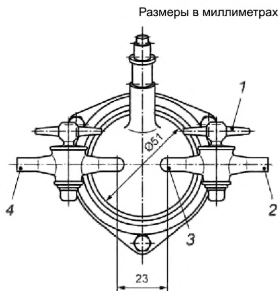
1 — запорный клапан; 2 — вход; 3 — трубка для подачи жидкости или газа; 4 — выход
