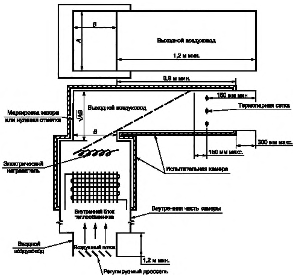
а) Схема для восходящего потока
