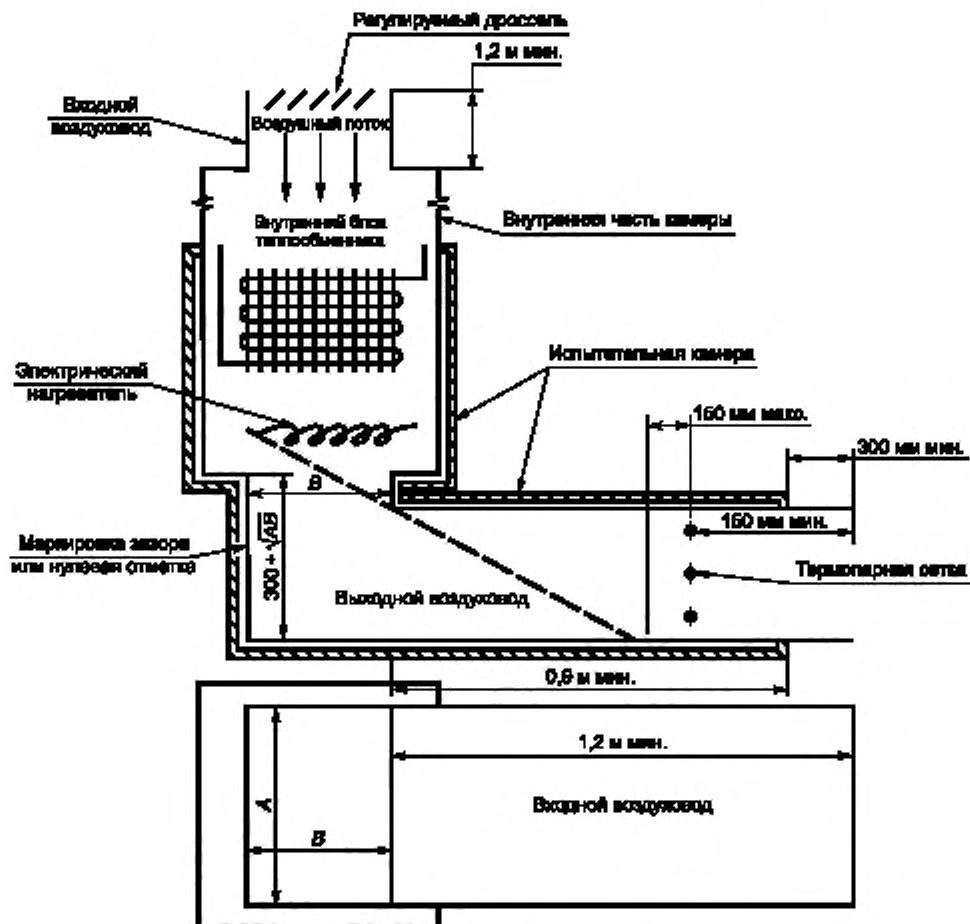
b) Схема для нисходящего потока
