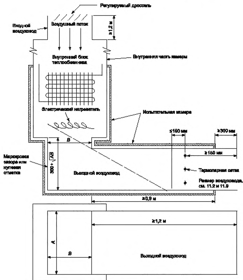
b) Схема для нисходящего потока
