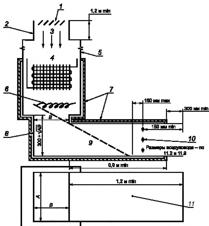
1 — регулирующий дроссель; 2 — входной воздуховод; 3 — воздушный поток; 4 — внутренний блок спиралей; 5 — внутренняя часть камеры; 6 — электрический нагреватель; 7 — испытательная камера; 8 — метка зазора или нулевая отметка; 9 — выходной воздуховод; 10 — термопарная сетка; 11 — выходной воздуховод
