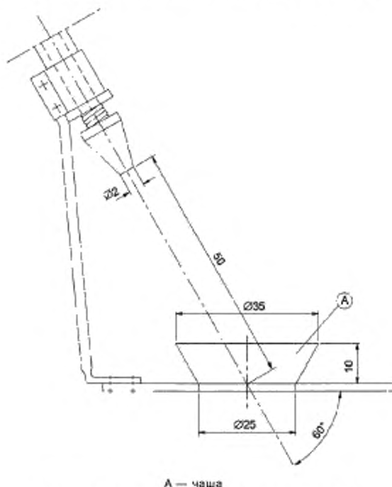
Рисунок 101 — Устройство для разбрызгивания
