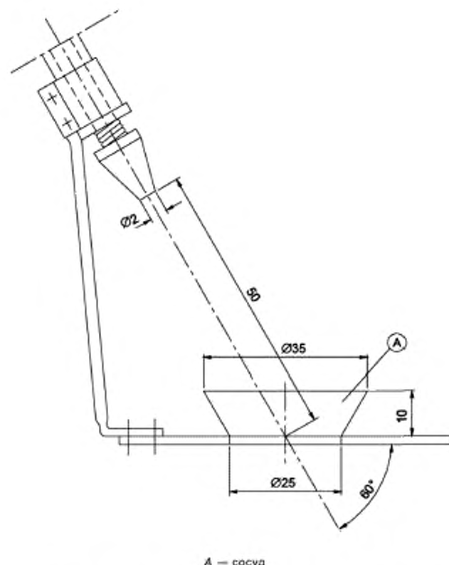
Рисунок 101 — Устройство для испытания обрызгиванием
