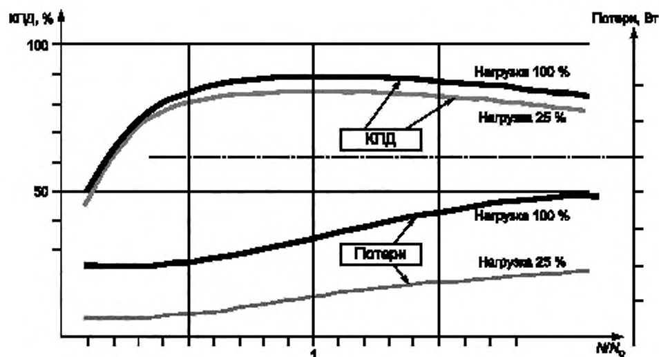
Рисунок 5 — Типовые кривые для КПД и потерь электропривода
