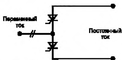
Пример однофазного моста Гретца
