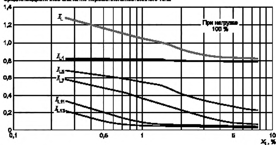
Рисунок В.9 — Входной гармонический ток
