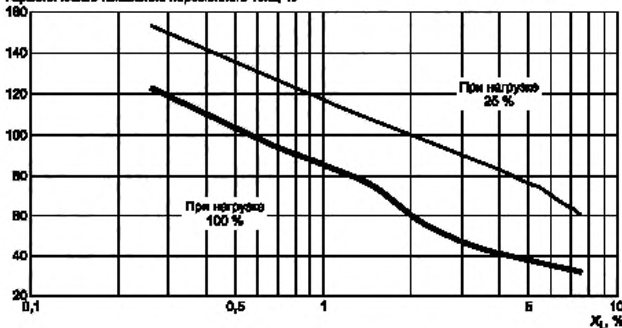
Рисунок В.10 — Искажение входного тока
