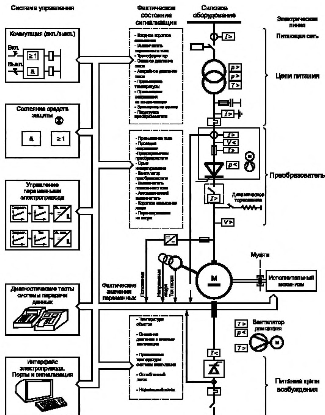
Рисунок 1 — Функциональная схема электропривода постоянного тока
