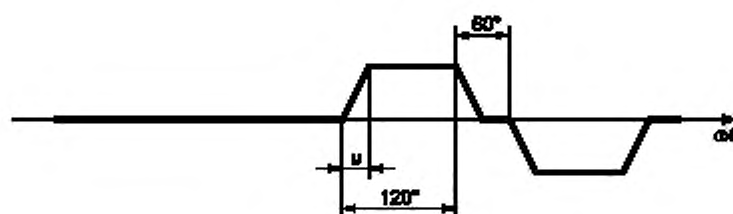
Рисунок В.3 — Трапецевидный ток питания
