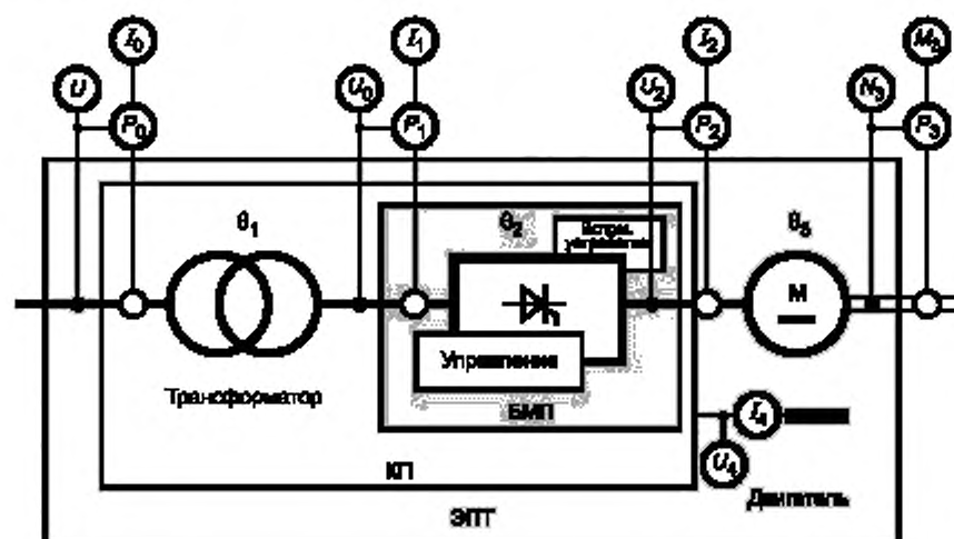
Рисунок 7 — Схема испытаний ЭПТ
