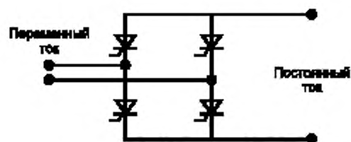
Пример однофазного моста Гретца
