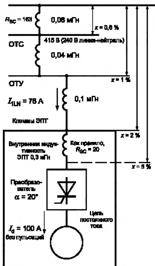
Рисунок В.11 — Пример простой структуры
