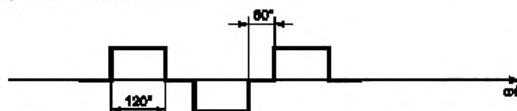
Рисунок В.2 — Прямоугольный ток питания
