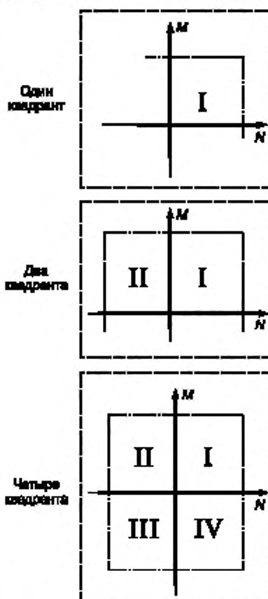
Рисунок 3 — Рабочие квадранты работы электропривода
