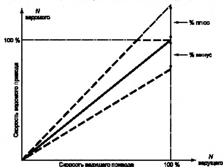
Рисунок D.6 — Система с ведущим/ведомым приводом
