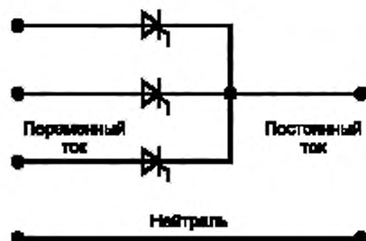
Пример трехфазного преобразователя
