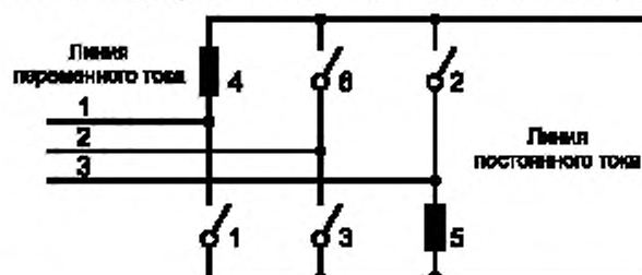
Рисунок В.12 — Трехфазный 6-пульсный мостовой преобразователь
