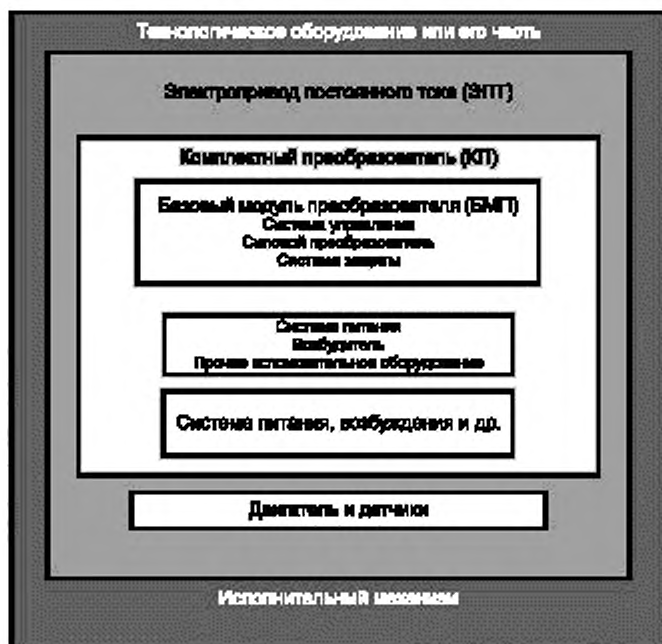
Рисунок 2 — Аппаратные составляющие ЭПТ
