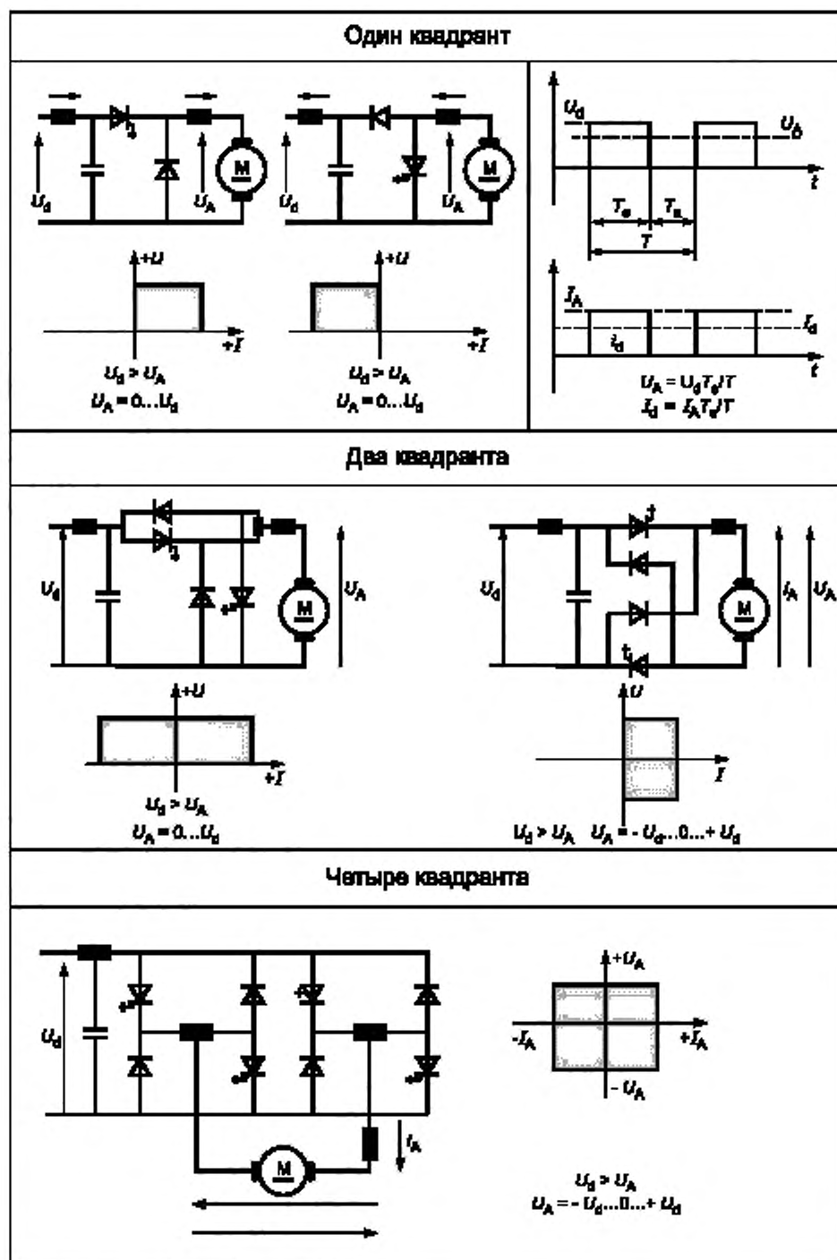
Рисунок F.2 — Преобразователи с внутренней коммутацией (прерыватели)
