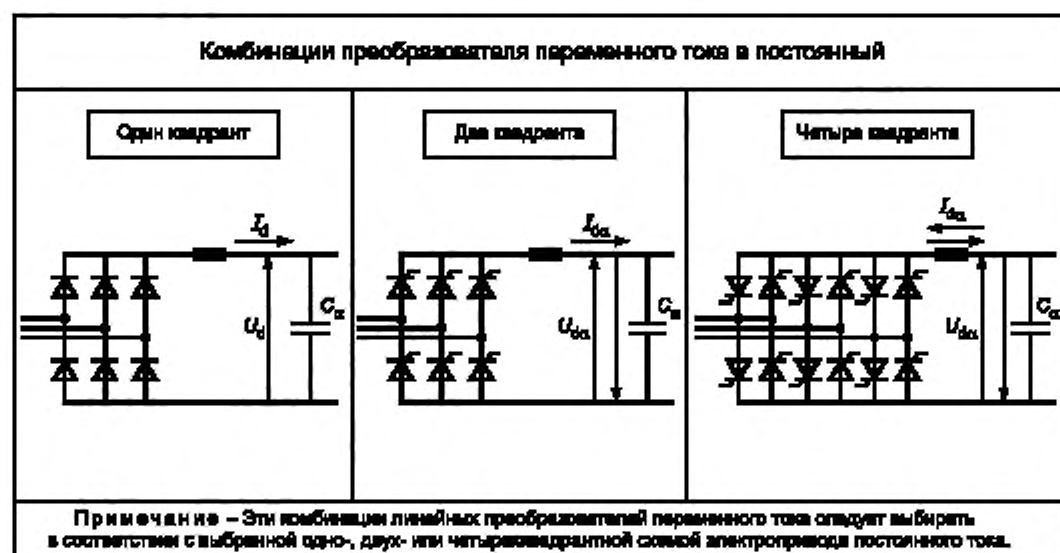
Рисунок F.4 — Обозначения схем прерывателей
