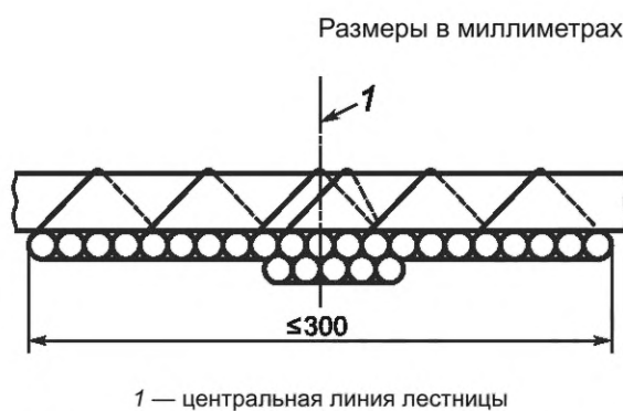
Рисунок 2 — Кабели, закрепленные на передней стороне лестницы без зазора (комплекты отрезков кабелей находятся в контакте)
