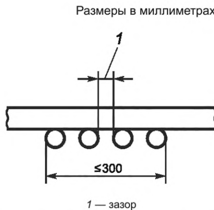
Рисунок 1 — Кабели, закрепленные на передней стороне лестницы с зазором
