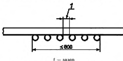
Рисунок 2 — Кабели, закрепленные на передней стороне широкой лестницы с зазором
