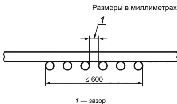
Рисунок 2 — Кабели, закрепленные на передней стороне широкой лестницы с зазором
