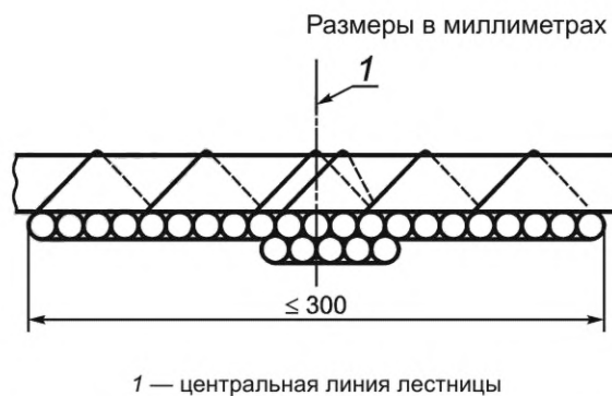
Рисунок 3 — Кабели, закрепленные на передней стороне стандартной лестницы без зазора (комплекты отрезков кабелей находятся в контакте)
