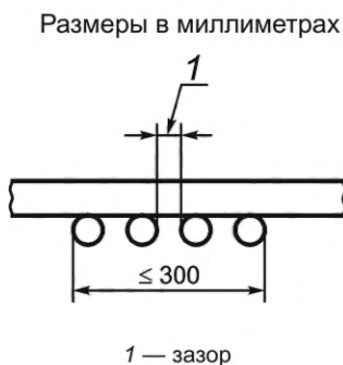
Рисунок 1 — Кабели, закрепленные на передней стороне стандартной лестницы с зазором
