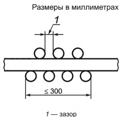
Рисунок 1 — Кабели, закрепленные на обеих сторонах лестницы с зазором (категория A F/R)
