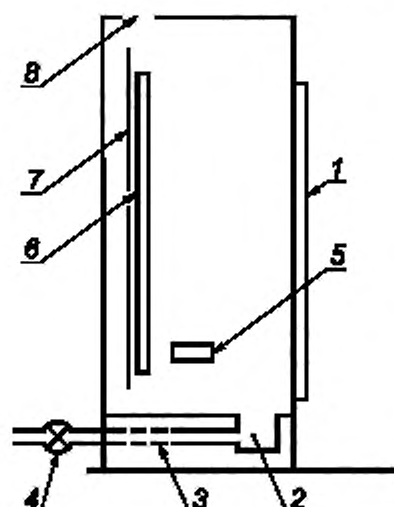
Рисунок 1б — Схематический вид сбоку испытательной камеры и устройства подачи воздуха
