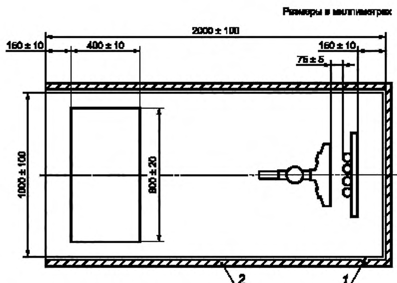
Рисунок 2 — Термоизоляция задней и боковых стенок испытательной камеры
