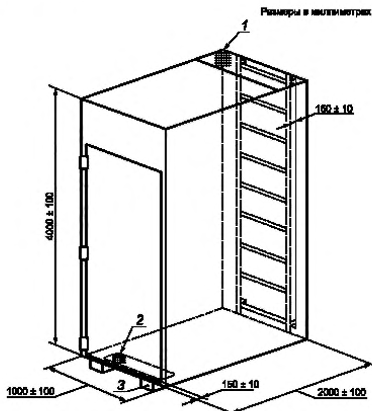
Рисунок 1а — Испытательная камера
