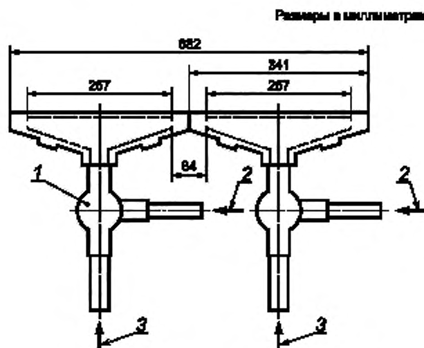
1 — смеситель Вентури для воздуха и газа; 2 — подача пропана; 3 — подача воздуха
