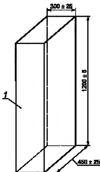
Рисунок 1 — Испытательная камера
