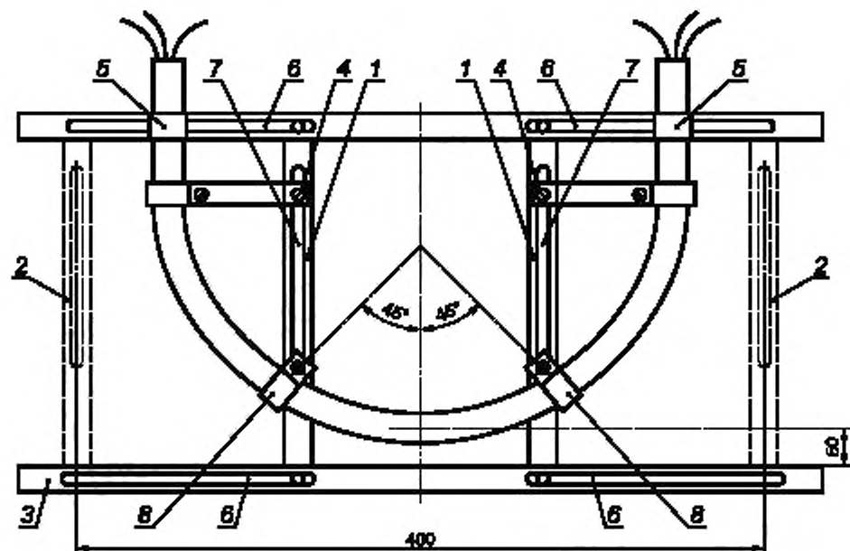
1 — отрегулированное положение вертикального элемента, 2 — исходное положение вертикального элемента, 3 — нижний горизонтальный элемент испытательной лестницы; 4 — дополнительный зажим для обеспечения дугообразной формы кабеля (если требуется); 5 — (U-образный хомут; 6 — прорезь для перемещения вертикального элемента. 7 — прорезь для крепления P-образного хомута; 8 — P-образный хомут
