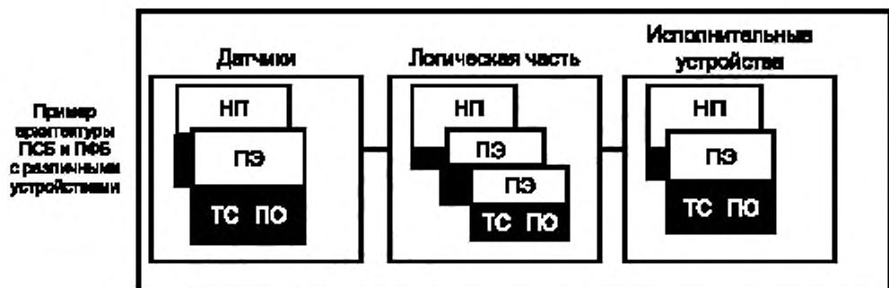
Рисунок 7 — Пример структуры ПСБ
