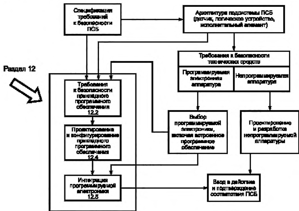
Рисунок 10 — Жизненный цикл безопасности прикладного ПО и его связь с жизненным циклом безопасности ПСУ
