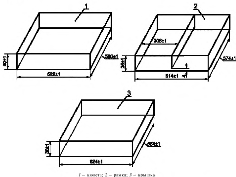
Рисунок 1 — Схема устройства для обработки образцов агрессивными средами
