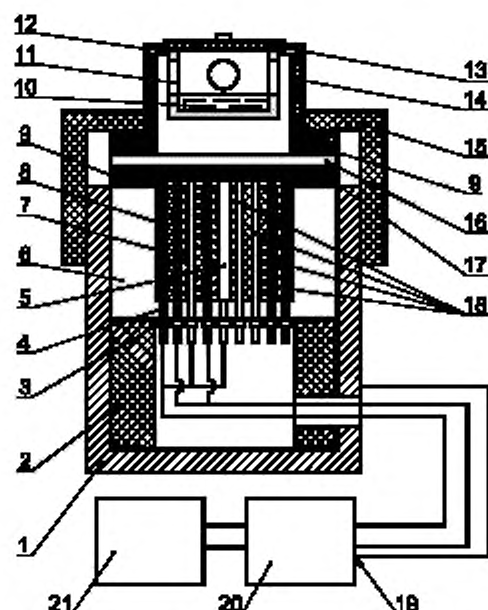
1 — корпус; 2 — подставка держателя; 3 — гайка крепления электродов; 4 — крепежный стержень электродов; 5 — центральный стержневой электрод; 6 — держатель кассеты; 7 — фторопластовая прокладка; 8 — кассета электродов; 9 — шайбы; 10 — жидкость; 11 — отверстия вкладыша; 12 — вкладыш; 13 — крышка; 14 — стакан; 15 — прижимная гайка; 16 — элементарная проба; 17 — прокладка из фильтровальной бумаги; 18 — кольцевые электроды; 19 — клемма «Экран» тераомметра; 20 — тераомметр; 21 — потенциометр
